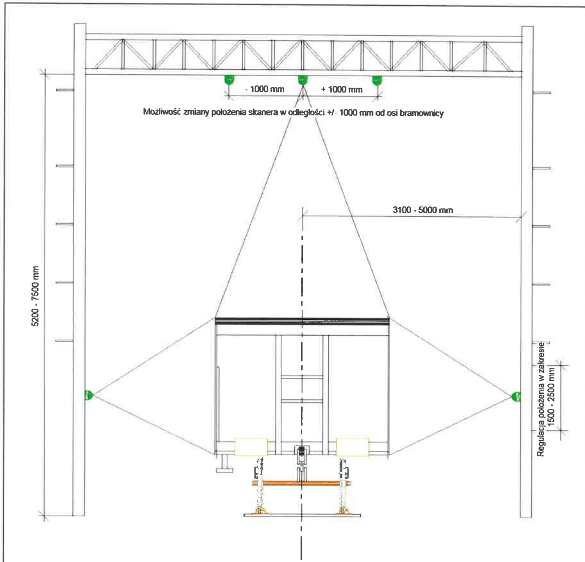
Rys. 2. Koncepcja rozmieszczenia uchwytów mocujących dla skanerów SICK LMS511-20100 PRO oraz skanera SICK LMS511-20100 PRO w obudowie sterującej. Zakres wymiarów konstrukcji bramownicy.
