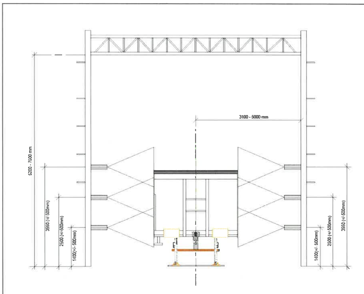
Rys. 1. Koncepcja rozmieszczenia uchwytych mocujących dla czujników do wysokorozdzielczej akwizycji obrazu w postaci 6 kamer w obudowach HEG 37K1A074. Zakres wymiarów konstrukcji bramownicy.
