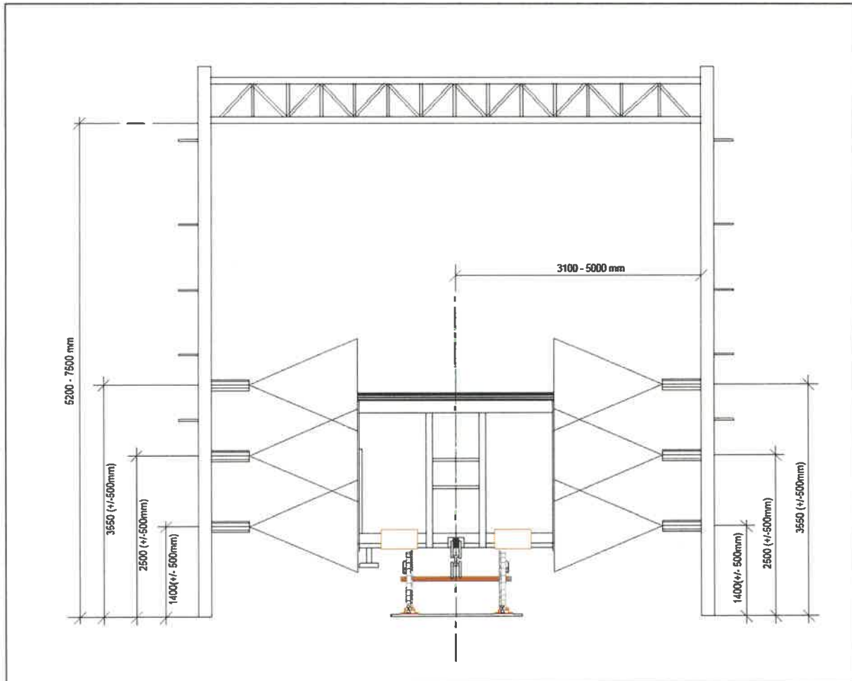
Rys. 1. Koncepcja rozmieszczenia uchwytów mocujących dla czujników do wysokorozdzielczej akwizycji obrazu w postaci 6 kamer w obudowach HEG 37K1A074. Zakres wymiarów konstrukcji bramownicy.
